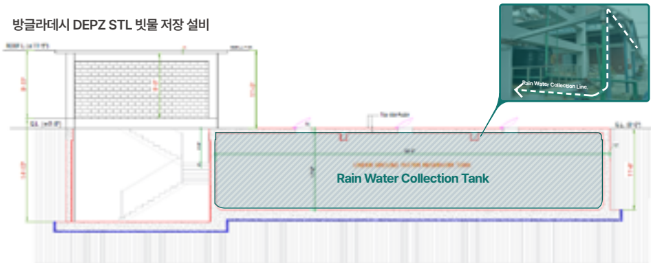
빗물 저장 설비 설계도
